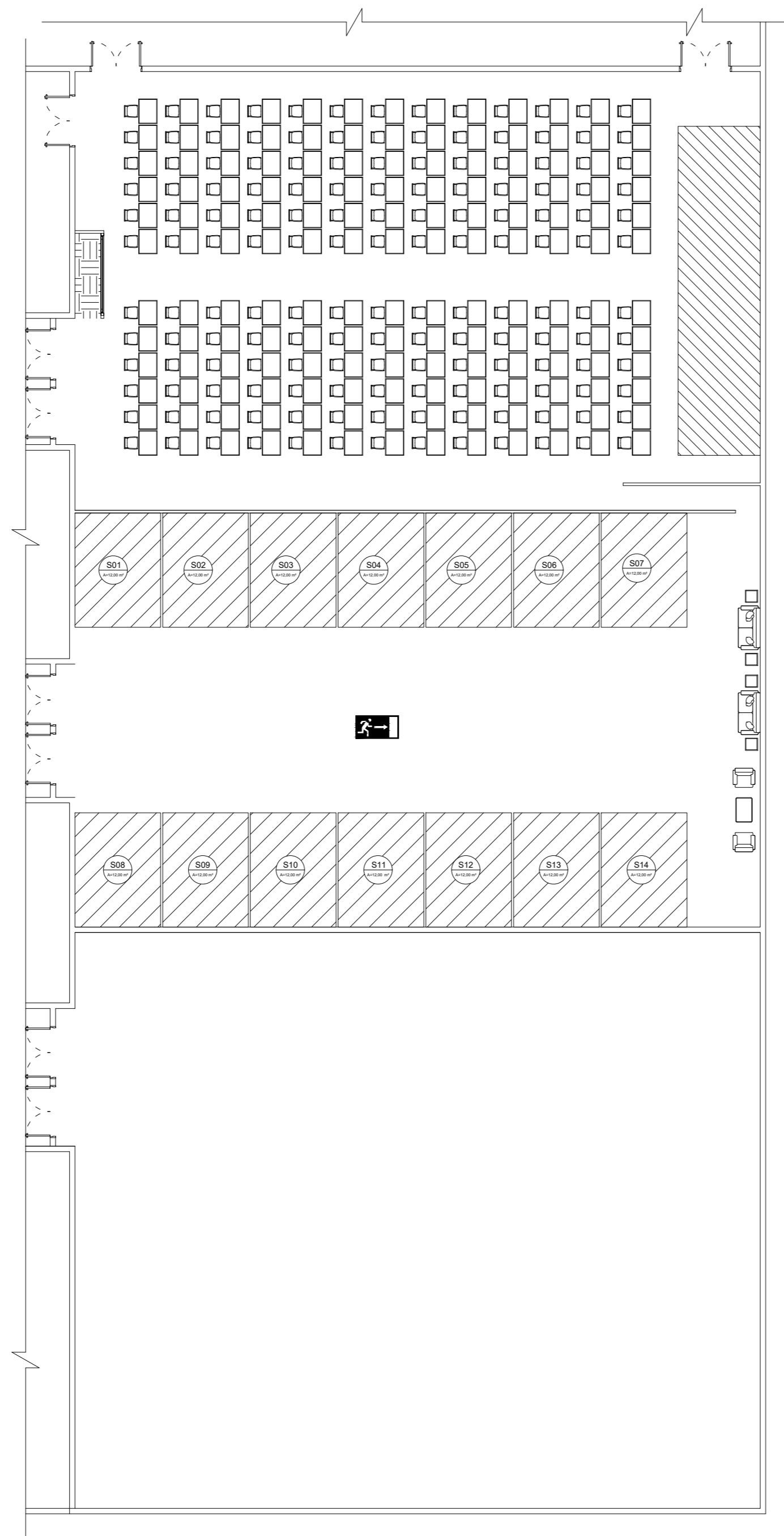
Opção - 1 ESC 1:150
